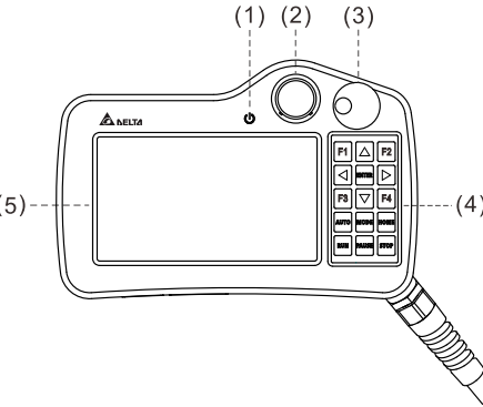
DOP-107HE42xZM / DOP-107HE46xZM (正面)
